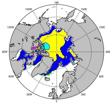
MPI
