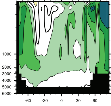
Kiel-ORCA zonal bias
