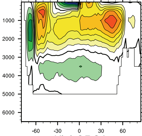
Kiel-ORCA
