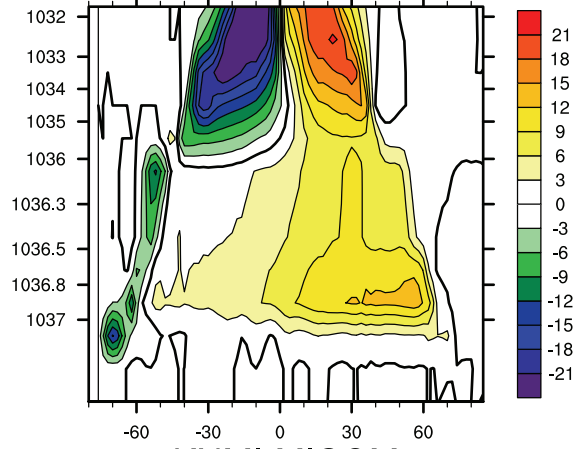
KNMI-MICOM
