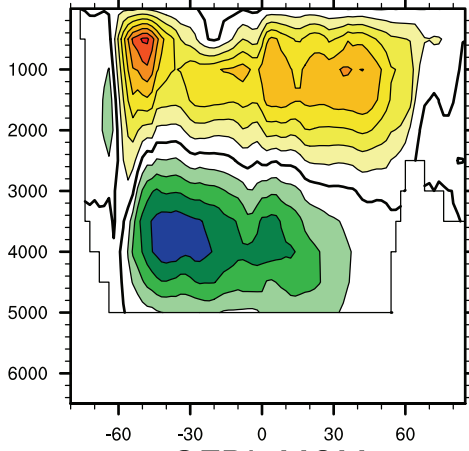
GFDL-MOM
