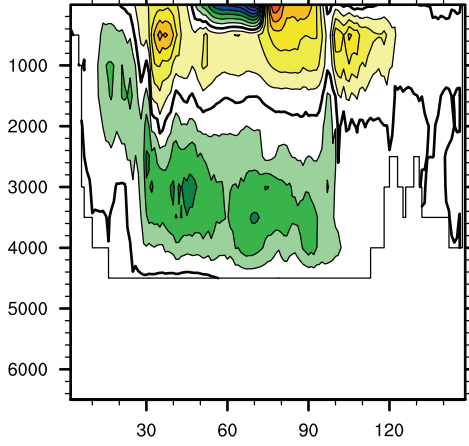
MPI
