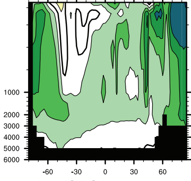
Kiel-ORCA zonal bias
